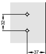
Placa de montaje en cruz
