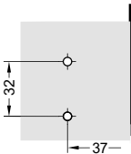
Placa de montaje
