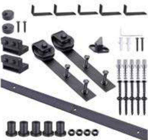
Elementos del kit
