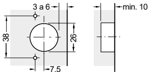
Medidas de taladro para la caja de la bisagra para atornillar
