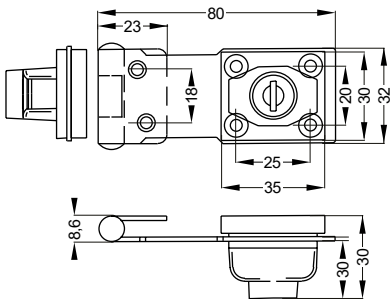
Detalle de mecanismo
