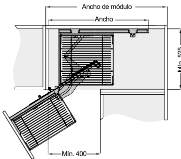
Apertura del lado derecho
