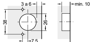
Medidas de taladro para la caja de la bisagra para atornillar
