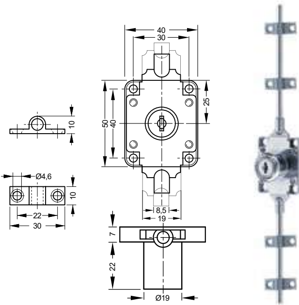
Plano de detalle
