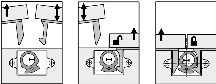
Detalle de mecanismo
