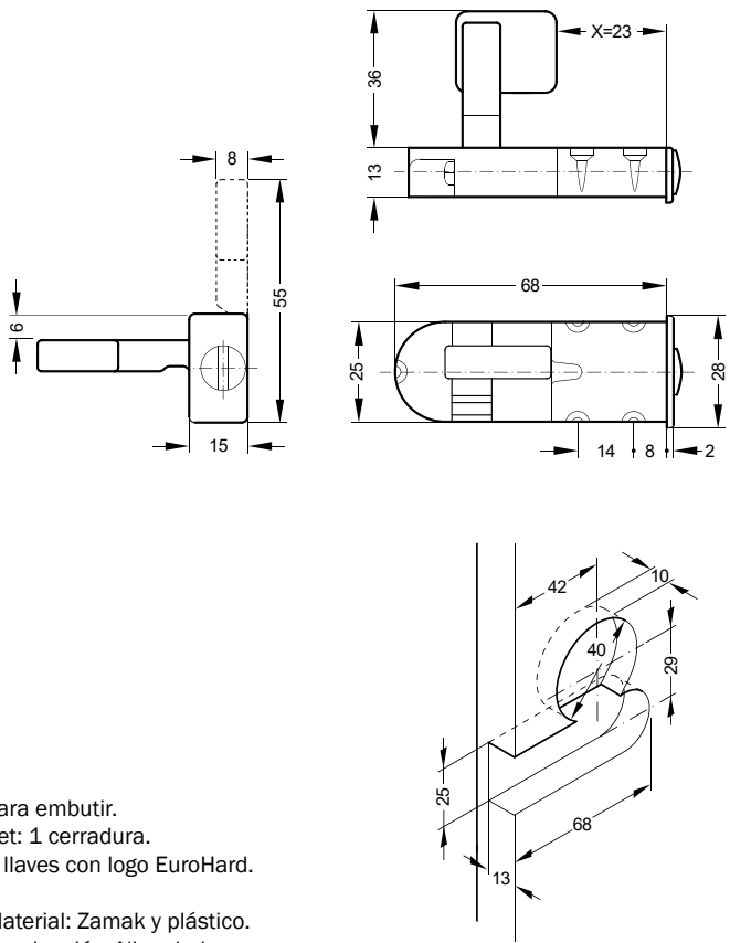
Plano de detalle
