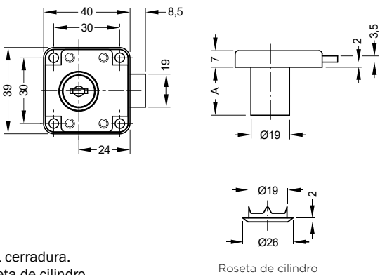
Plano de detalle
