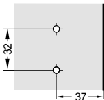
Placa de montaje en cruz
