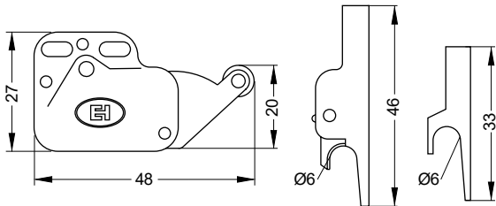
Plano de montaje
