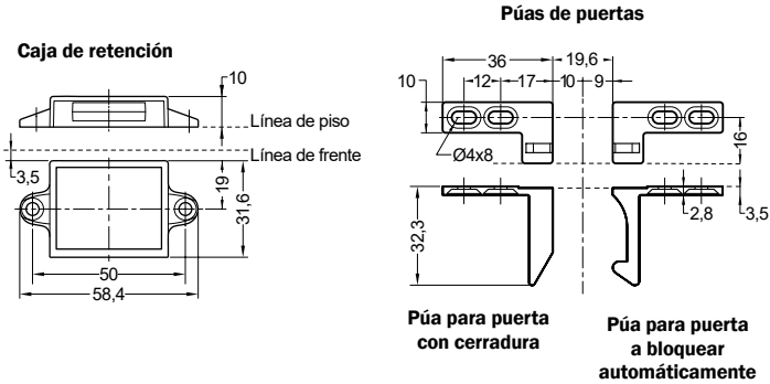
Detalle de mecanismo
