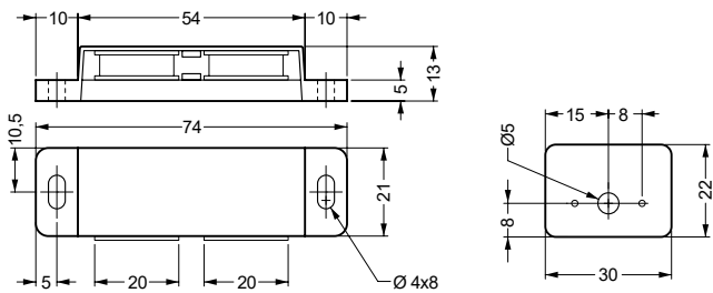
Plano de detalle
