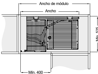
Apertura del lado izquierdo
