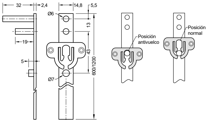
Varilla de cierre
