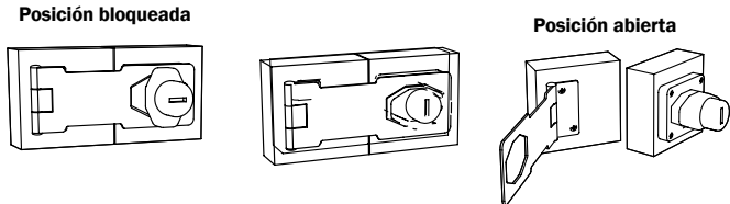
Detalle de mecanismo
