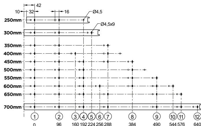
Perforaciones para lateral de cajón
