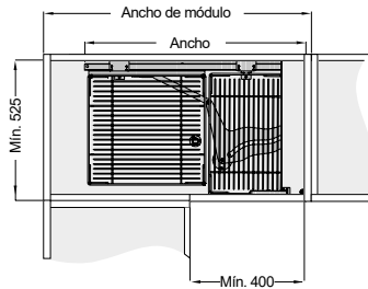
Apertura del lado derecho
