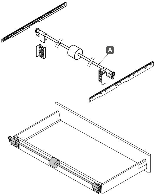
Plano de detalle
