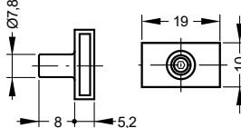
Púas para varilla anti caída
