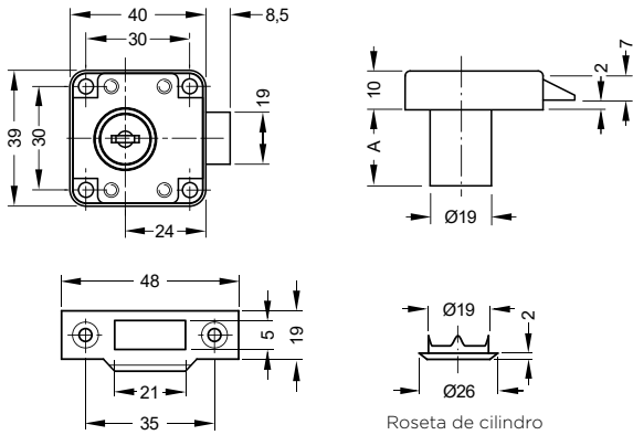
Plano de detalle
