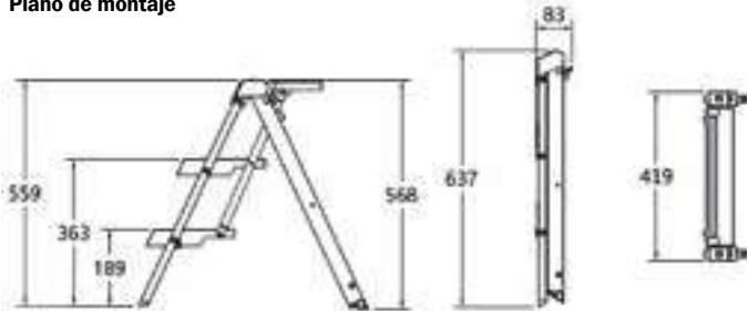
Plano de montaje
